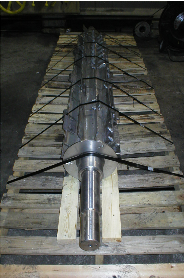
Rotor for Voith RS2B Rejectsorter
